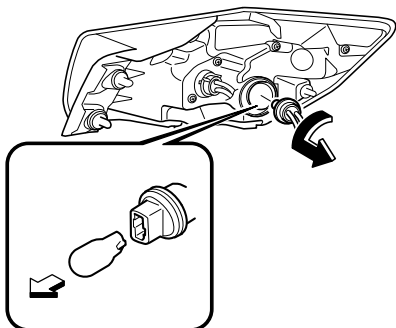
Feux de position arrière
