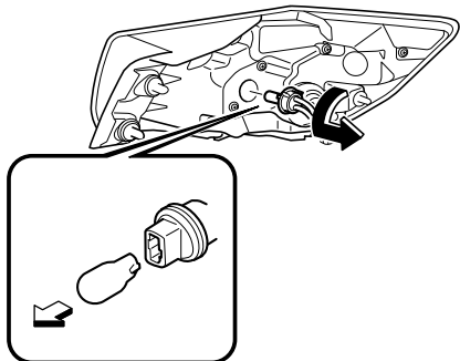
Feux de freinage/Feux arrière
