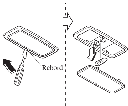
Eclairages au pavillon (arrière)
