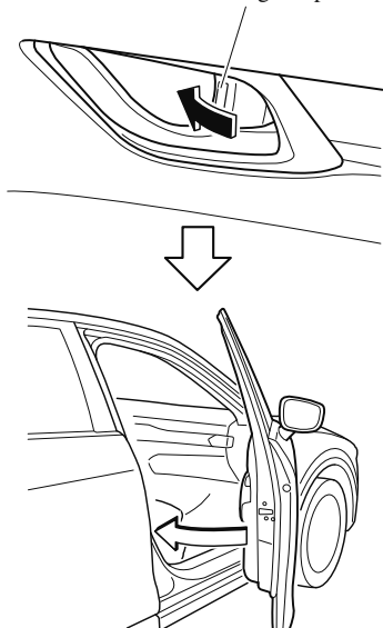
Commande de verrouillage de portière
