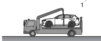
1. Chariots porte-roues
