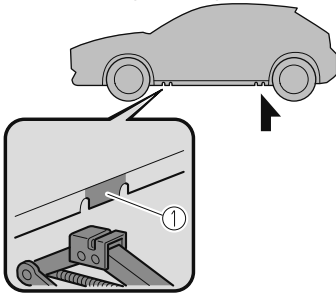
1. Position de levage
