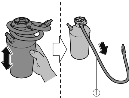
1. Tube d'injection
