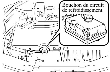
Réservoir de liquide de refroidissement
