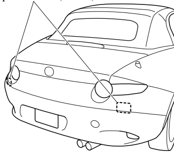
Capteurs radar (arrière)
